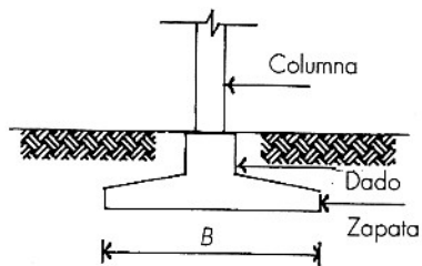
c) Zapata aislada y/o corrida
