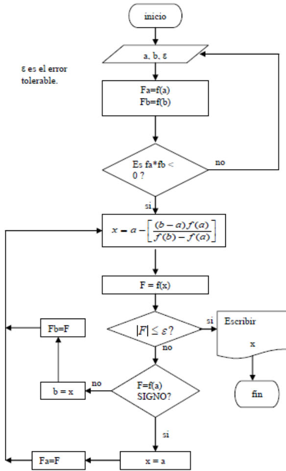
Fig. D.3.3 Diagrama de flujo: método FALSA POSICION
