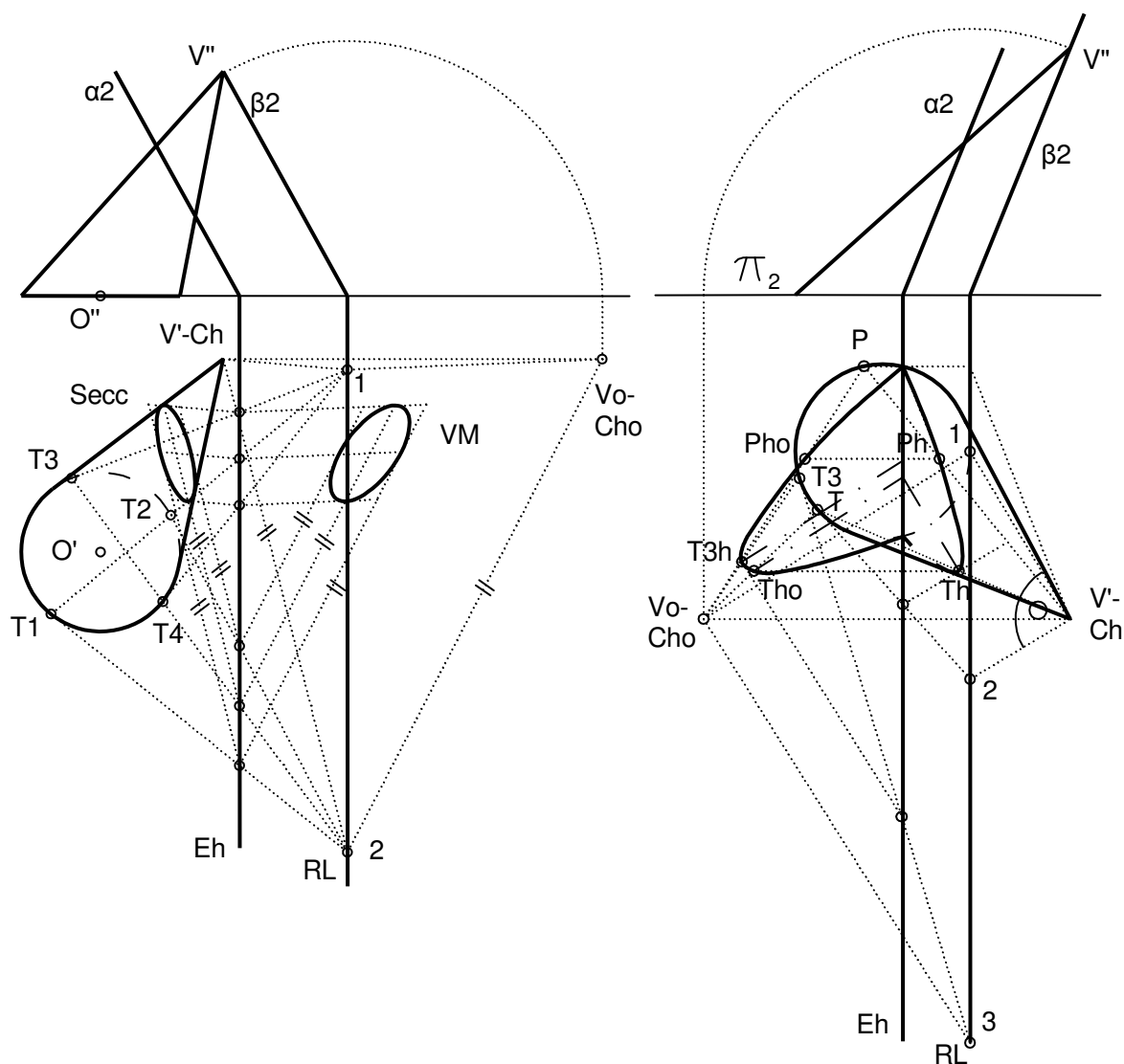
Figura 16: Sección plana del cono: Elipse y Parábola.
