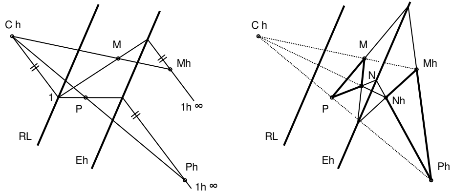
Figura 12: Homología plana.
