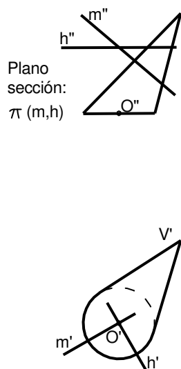
Figura 5: Sección con plano \pi(m,h) y desarrollo de un cono y transformada de la sección.
